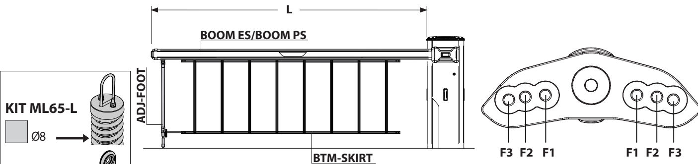
L (m) LUNGHEZZA BARRA / BOOM LENGTH / LONGUEUR BARRE / STANGENLÄNGE / LONGITUD DE LA BARRA / LENGTE STANG
